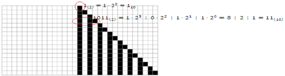
Slika 3.9: Generiranje Jacobsthalova niza pomoću elementarnih staničnih automata.
