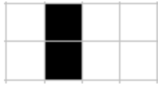
Slika 3.4: Prva ćelija drugoga retka rešetke elementarnih staničnih automata.
